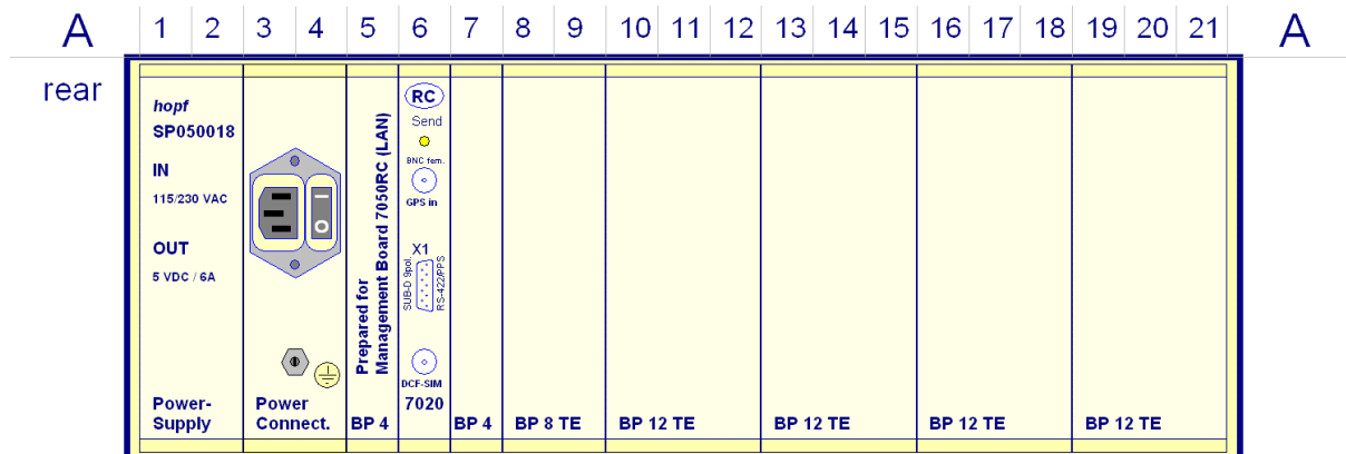
Beispielsystem, Rückseite/Einschubseite:
